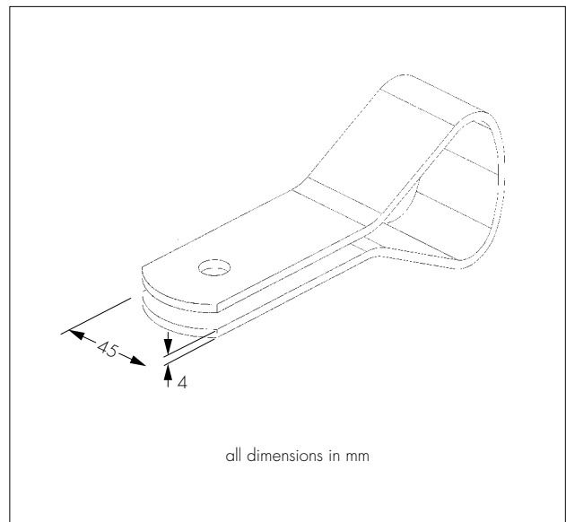
Figure 2 Panel Lug
